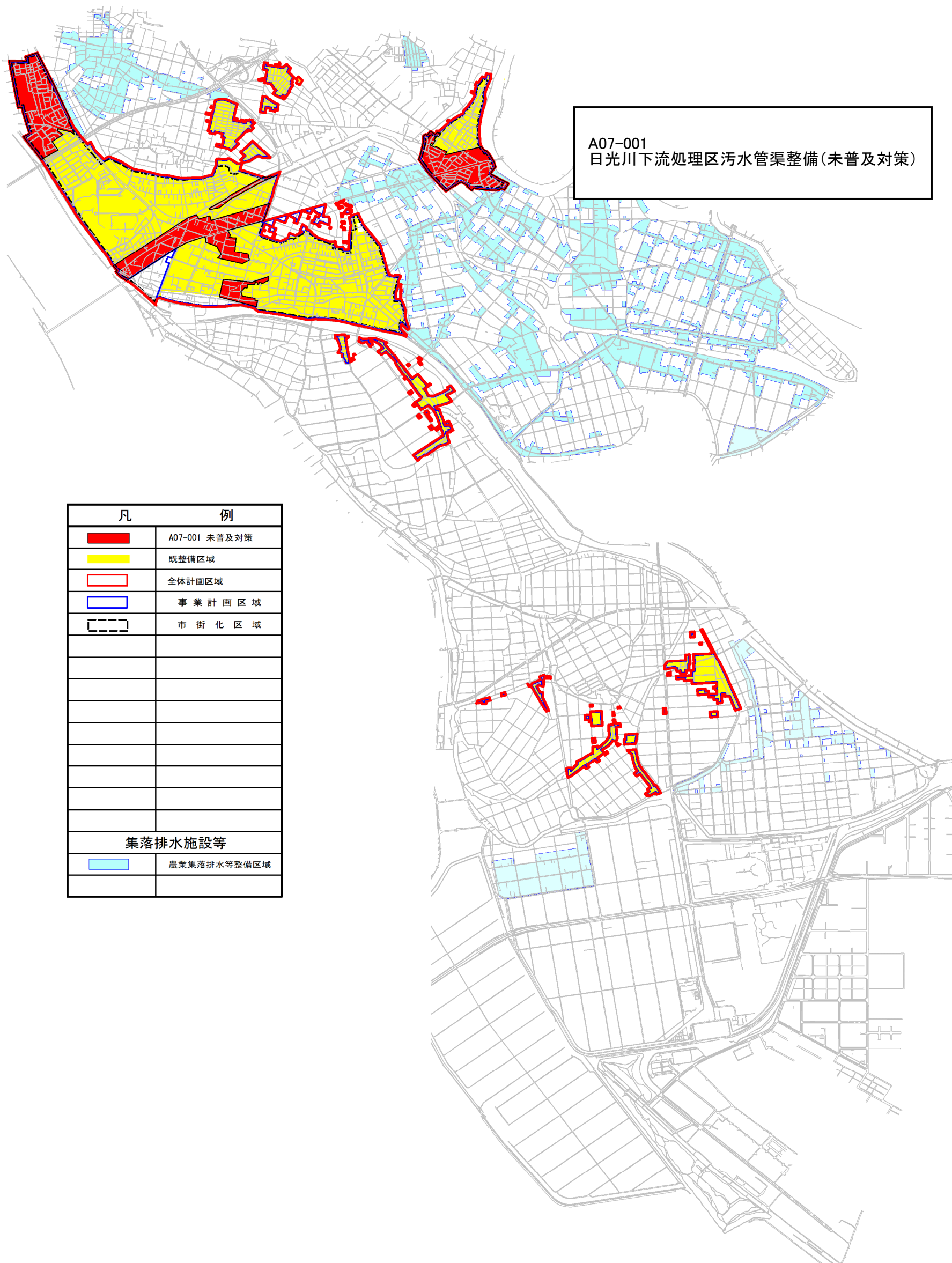
弥富市下水道計画一般図（污水）
