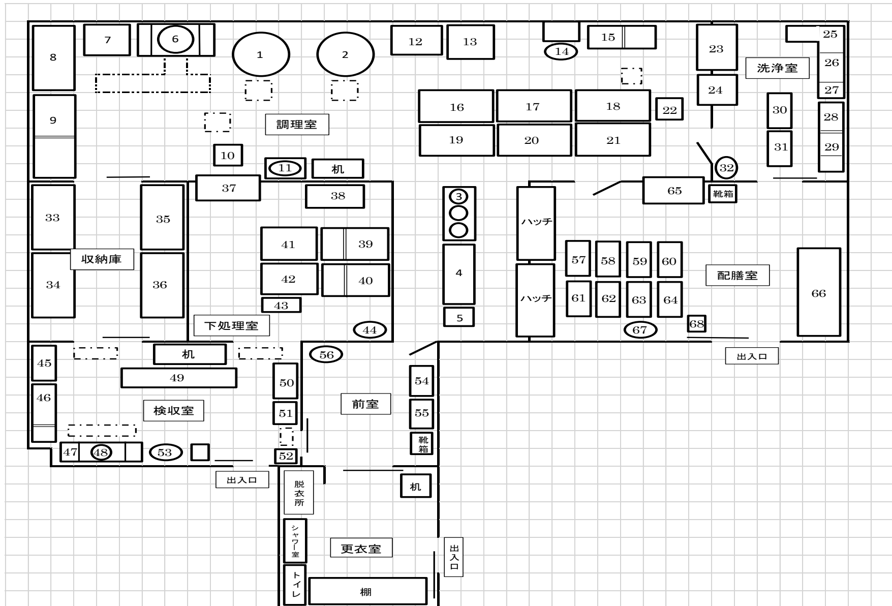
白鳥保育所 調理室配置図 R 7. 8 現在
